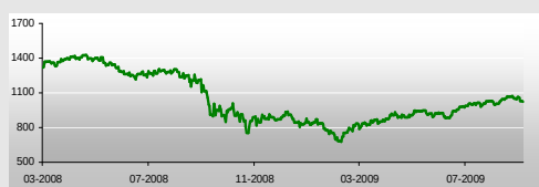
S&amp;P 500
