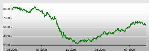
Miedź
